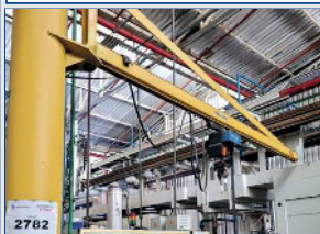
PÓRTICO C/BRAÇO GIRATÓRIO
