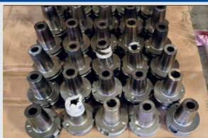
MANDRIS PARA FERRAMENTAS DIVs
